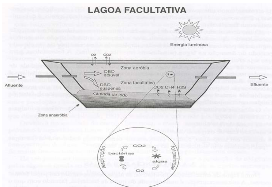
Fig. 2.2. Esquema simplificado de uma lagoa facultativa
