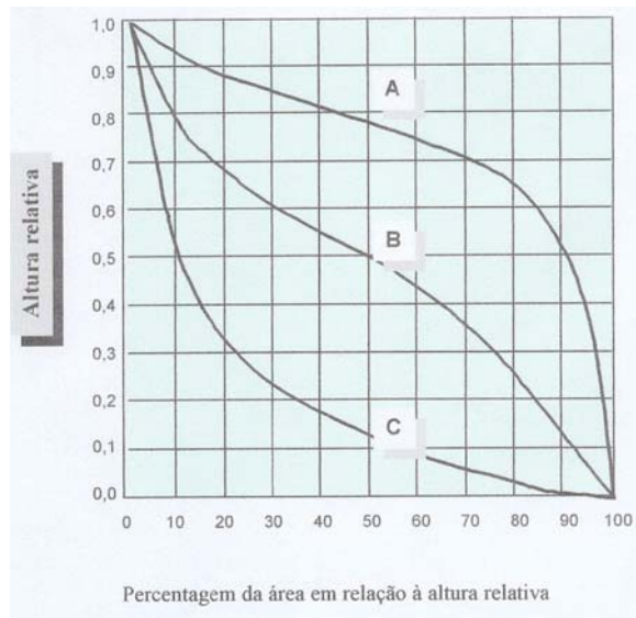
Fig- 04. Curvas hipsométricas/características do ciclo de erosão
