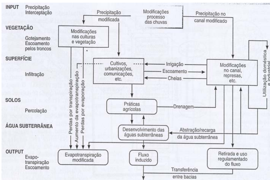
FIG. 01 - Modelo caracterizando o ciclo hidrológico em bacias hidrográficas, assinalando os fluxos e armazenagens e identificando influências artificiais conforme (LEWIN, 1995).
